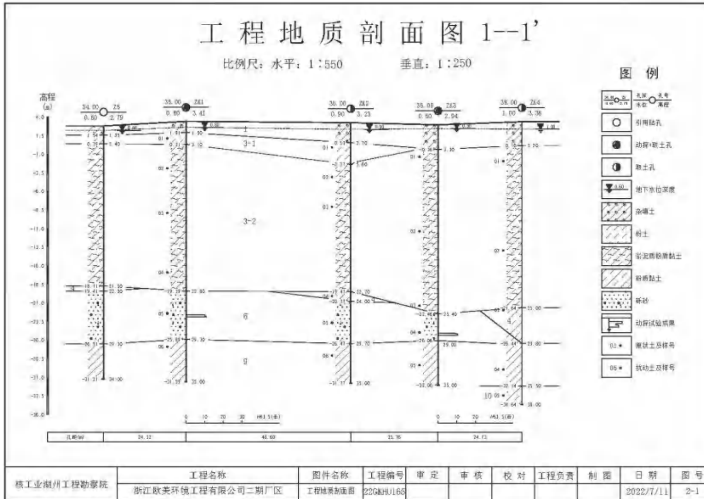
图 3.1-2 地质剖面图
