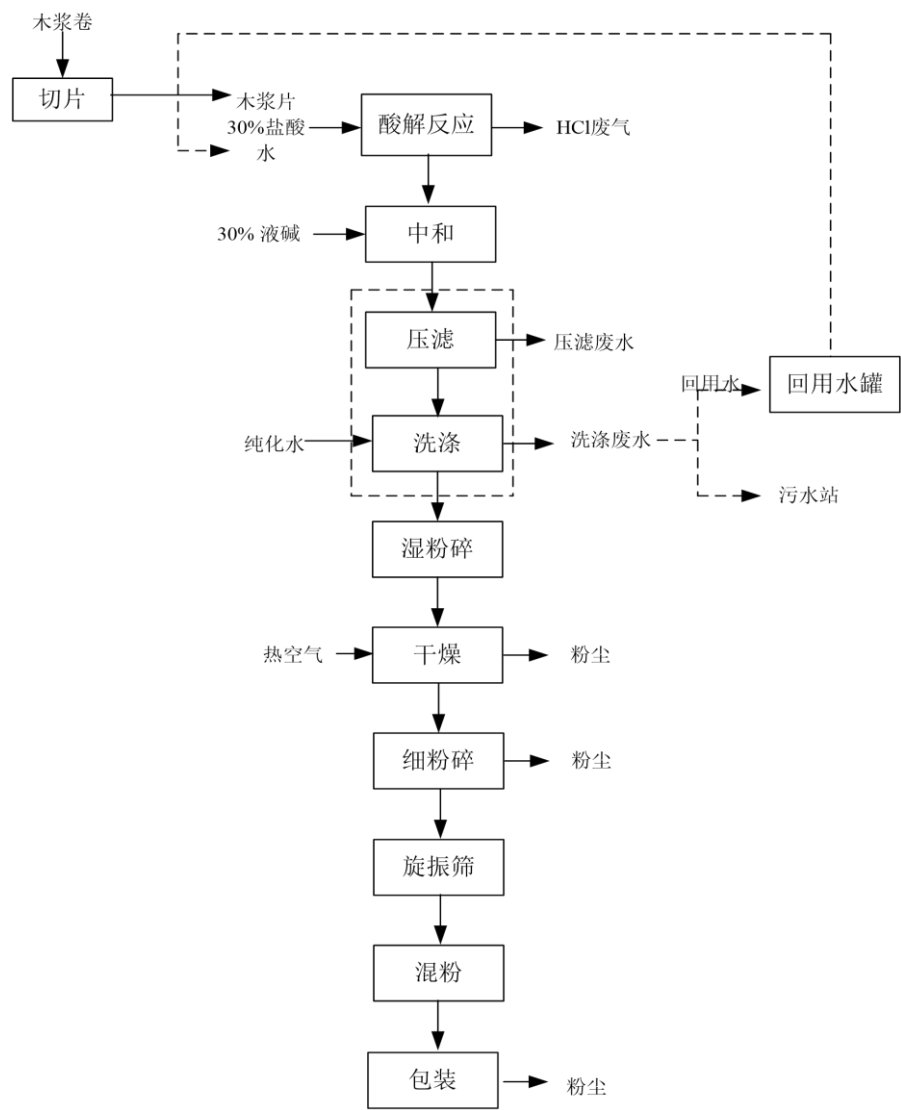
图 4.1-3 微晶纤维素生产工艺流程图
